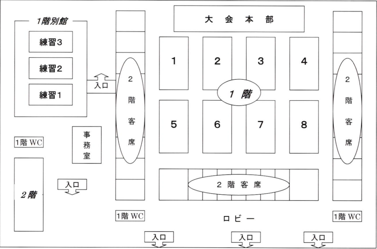
宮崎県体育館見取図
